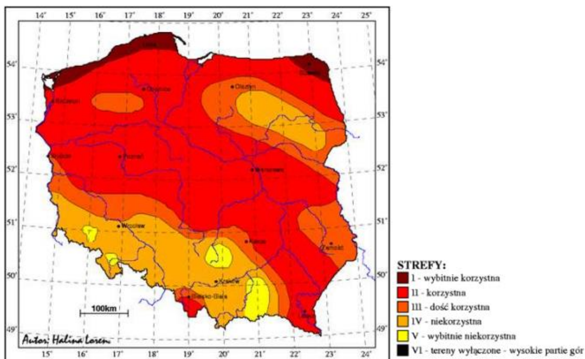
Rysunek 42. Strefy energetyczne wiatru w Polsce wg H. Lorenc [1996]
