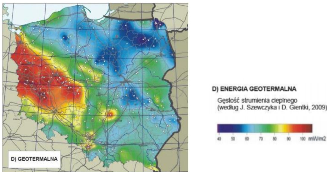
Rysunek 43. Zasoby energii geotermalnej w Polsce (źródło: Koncepcja Przestrzennego Zagospodarowania Kraju )
