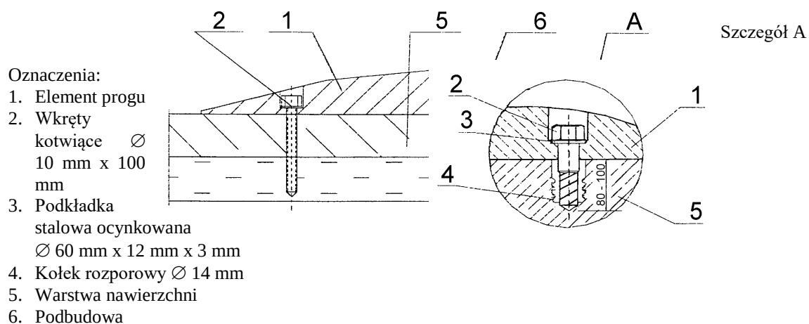
Rys. 4. Przykład umocowienia progu do nawierzchni jezdni
