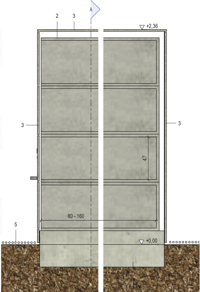
Przekrój B-B
