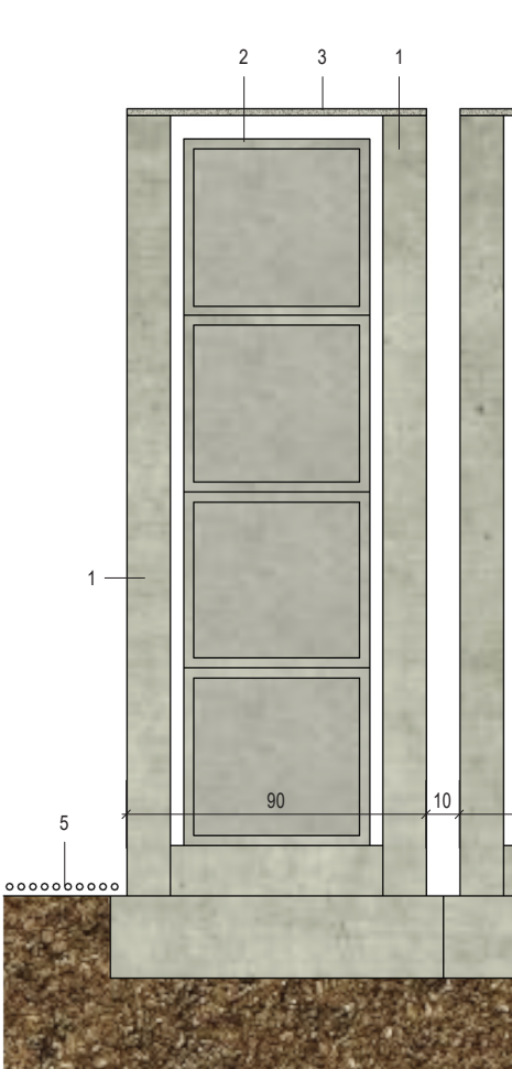
Przekrój A-A
