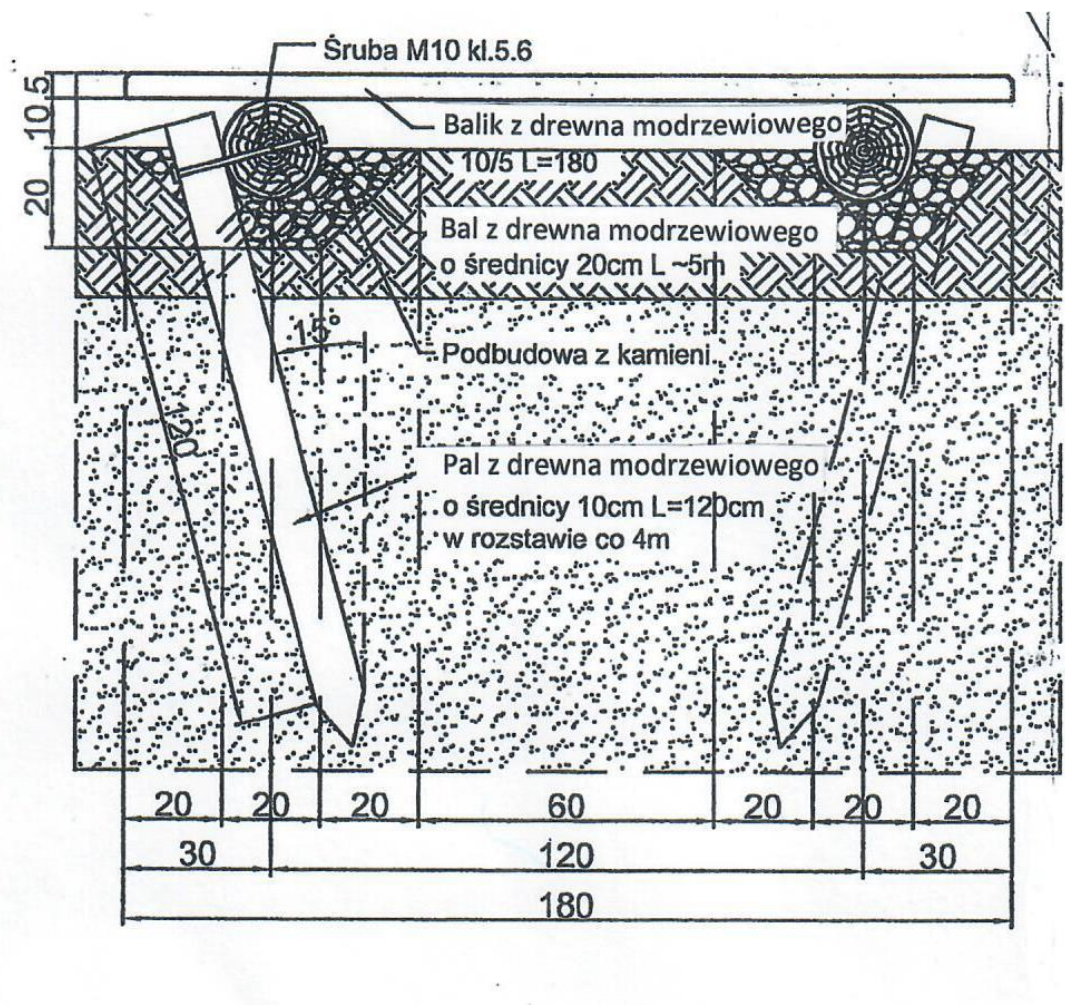
Rys. nr 3. Przekrój poprzeczny istniejącej „kładki”
